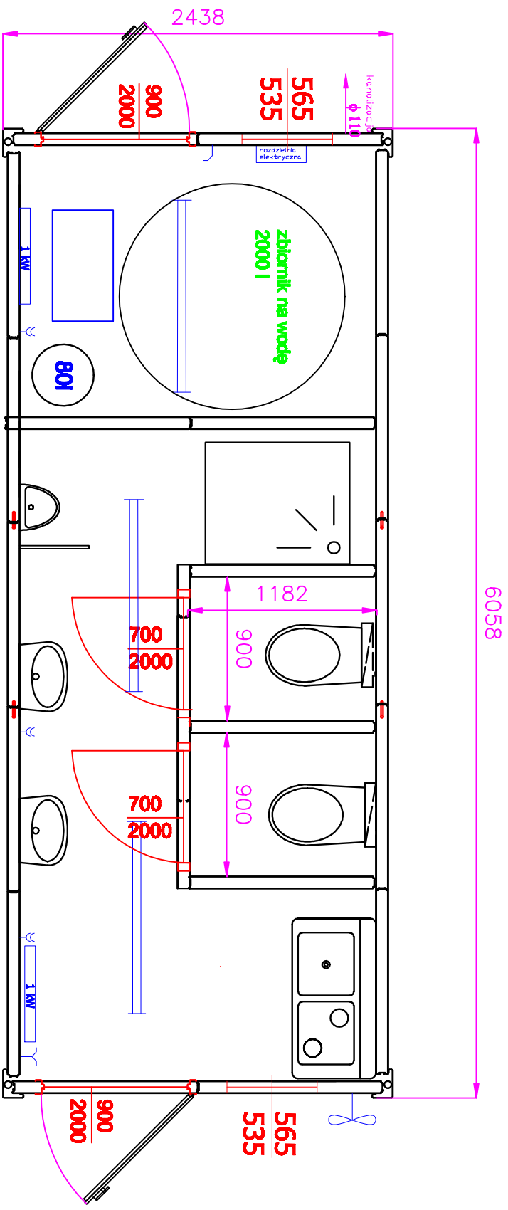
rys. 1 kontener sanitarny
